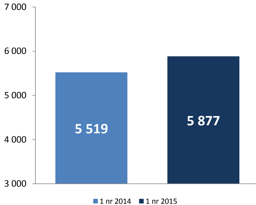
Динамика поступления заявок, шт.
